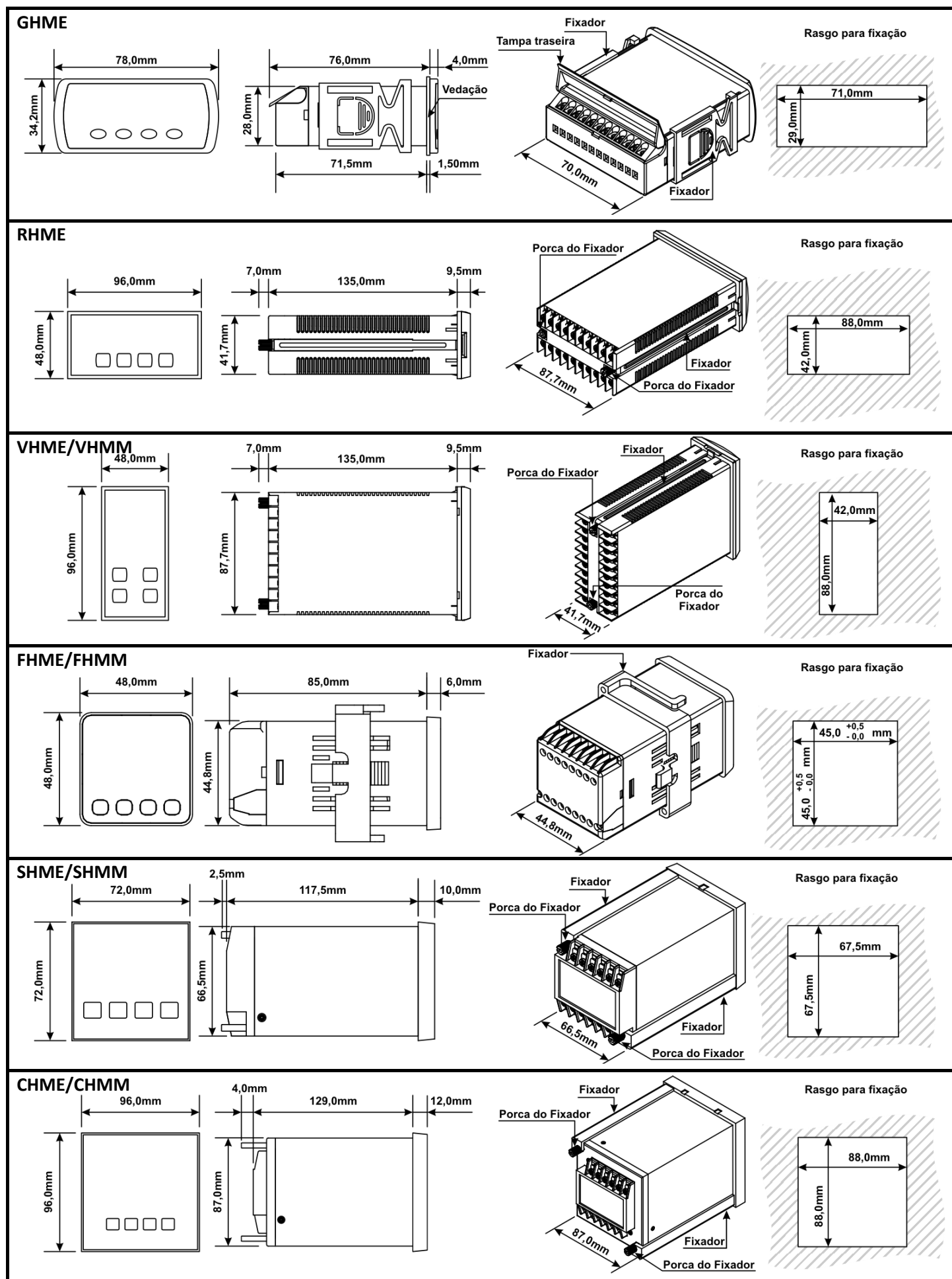
Figura 3 Dimensões das caixas.
