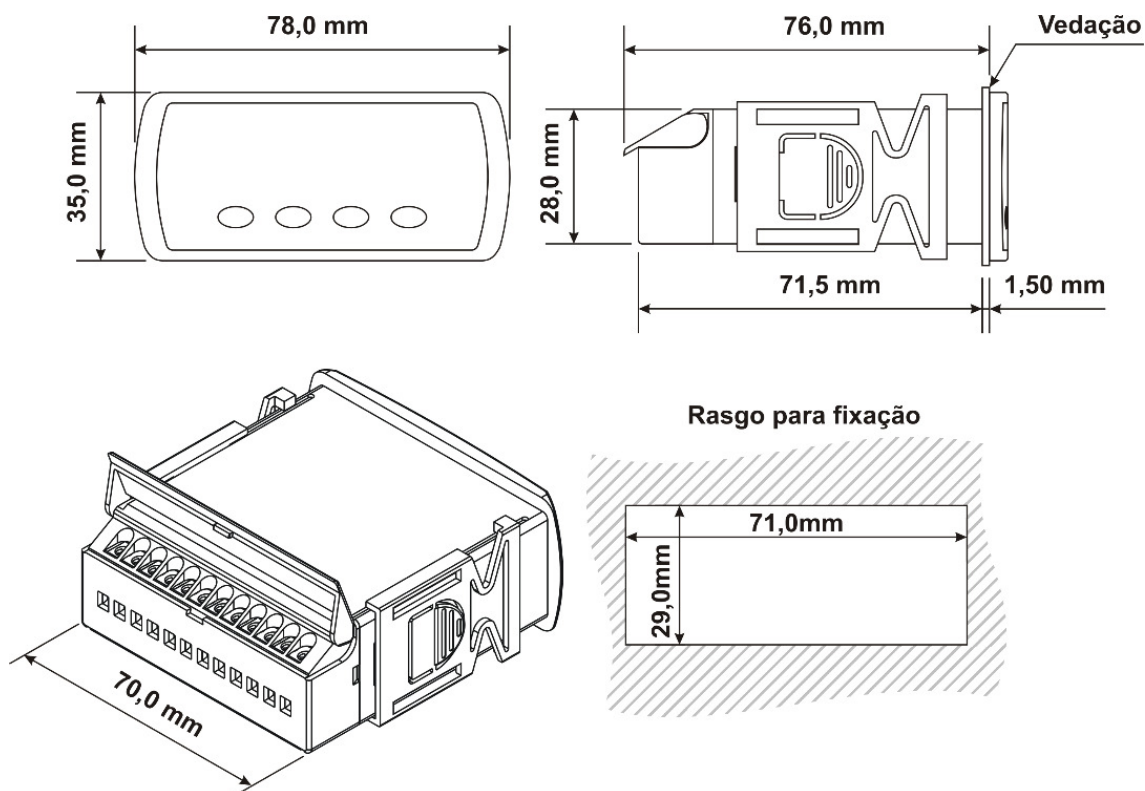
Figura 3 Dimensões.
