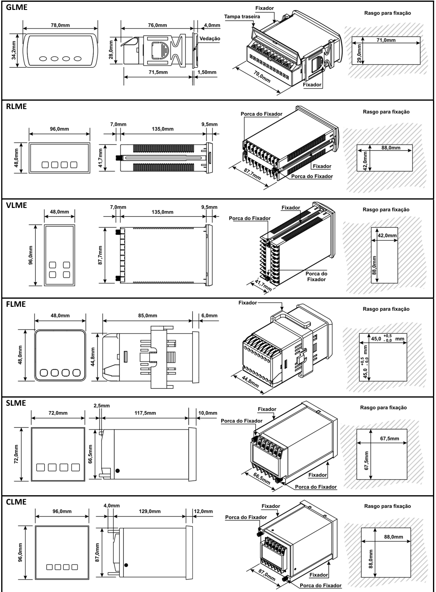
Figura 3 Dimensões da caixas.
