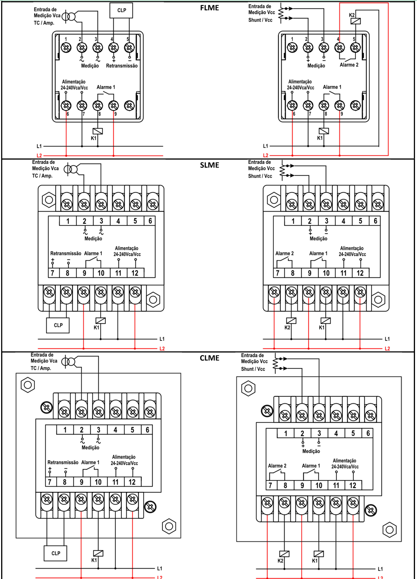
Esquema 1 Exemplo de ligação.
