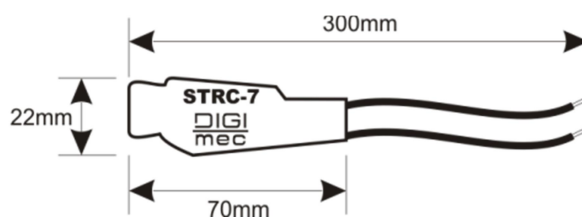
Figura 4 Esquema supressor de ruído elétrico e dimensões.
