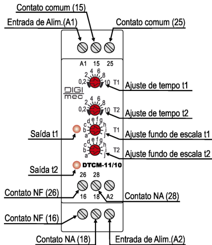
DTCM-11/10 - saída 2 [(25/26)-NF(25/28)-NA] simultânea com saída 1
