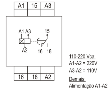
JTCM-1/10 e DTCM-1/10
