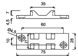
Adaptador para caixas D, fixação por parafusos (opcional).
