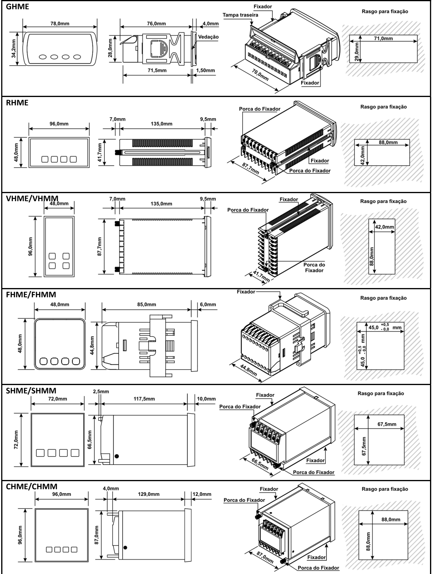
Figura 7 Dimensões da caixas.
