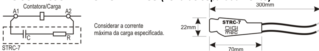
Figura 8 Esquema supressor de ruído elétrico e dimensões.
