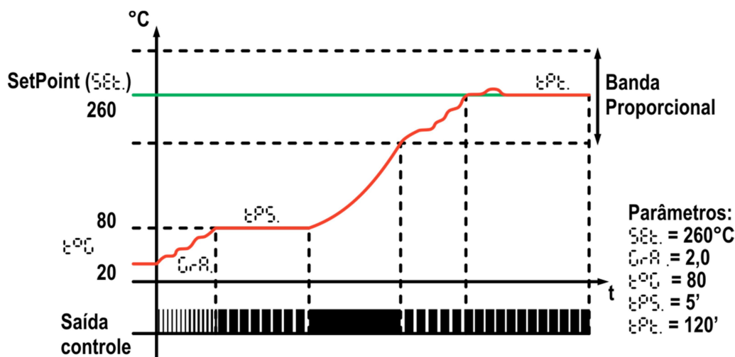
Figura 6 Exemplo de funcionamento do soft-start
